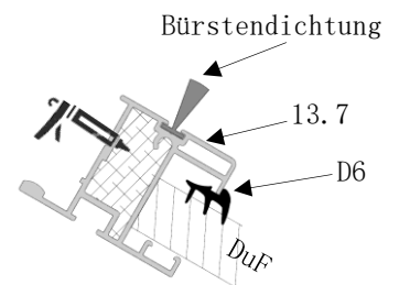
Schnittdarstellung
