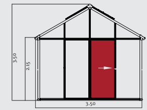
Alternativ: Einzelschiebetüren Türbreite: ca. 0,80 m
