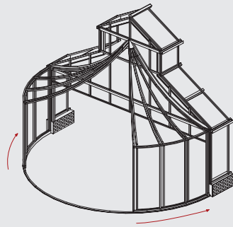
Giebelvorbau, inkl. verschiebbarem Dach
