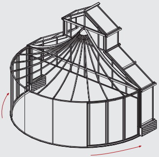
Giebelvorbau mit festem Dach, – Seitenelemente verschiebbar –
