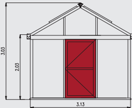
Standard: Drehtüren mit Drücker und Profilzylinder Türbreite: ca. 1,00 m
