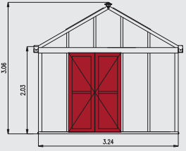
Standard: Doppeldrehtüren Türbreite: ca. 1,20 m
