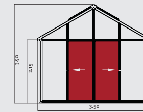
Standard: Doppelschiebetüren Türbreite: ca. 1,65 m
